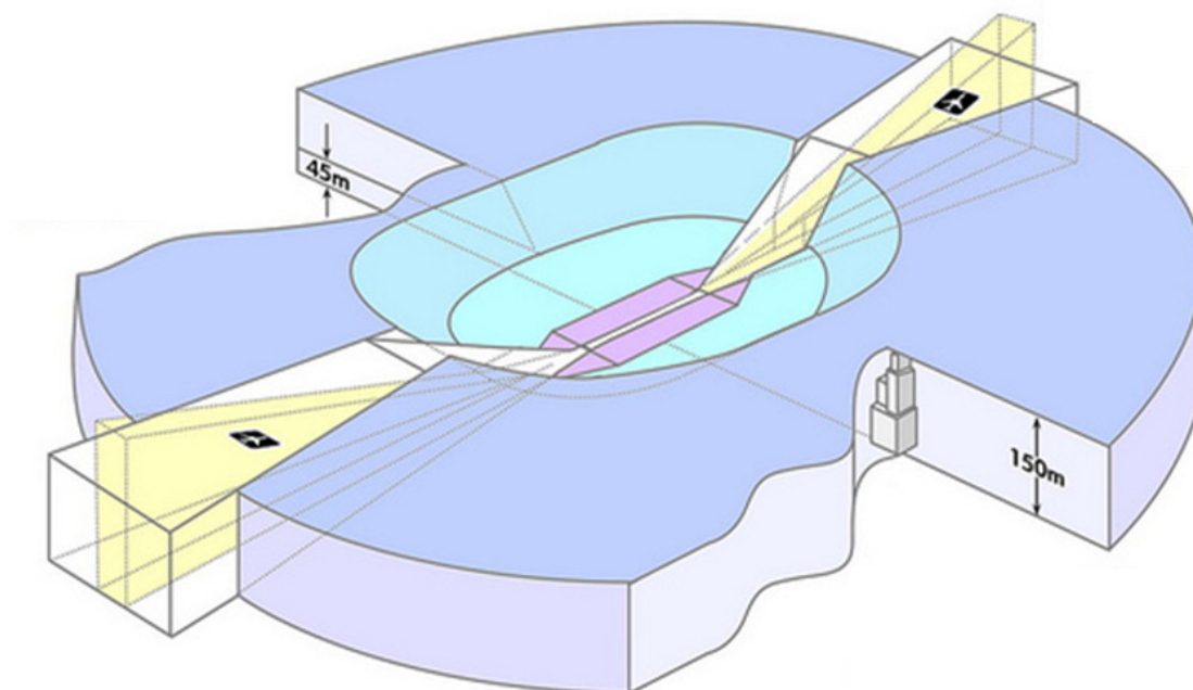
Figuur 2.2. Schematische weergave van de wettelijke hoogtebeperkingen rondom luchthavens
