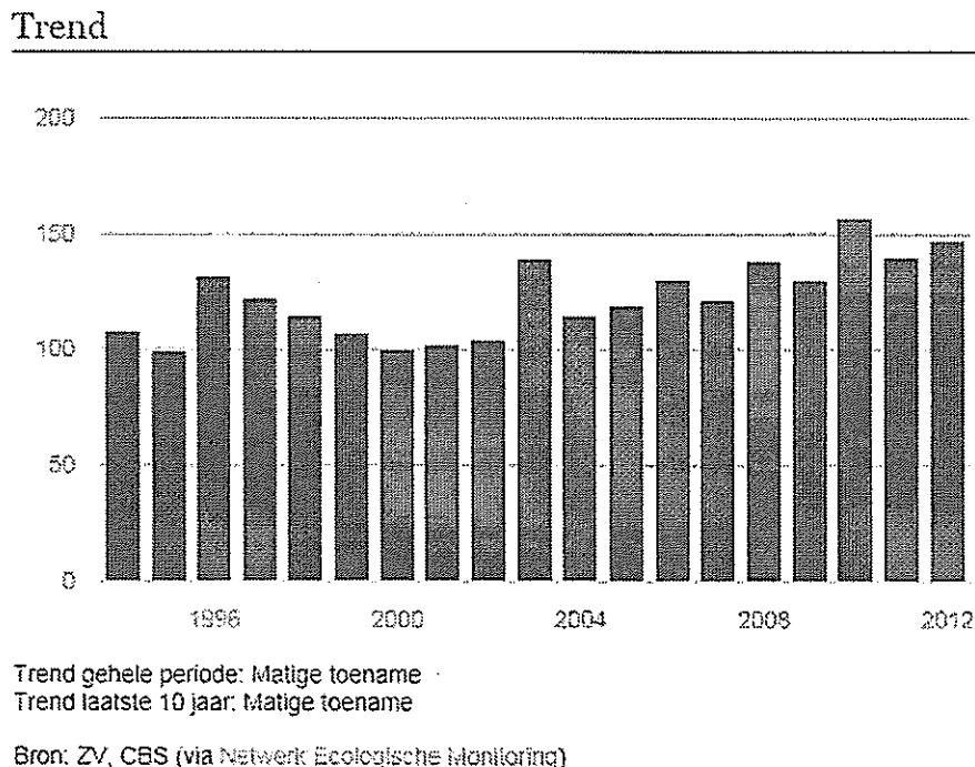
Figuur 1: Landelijke trend van het ree
