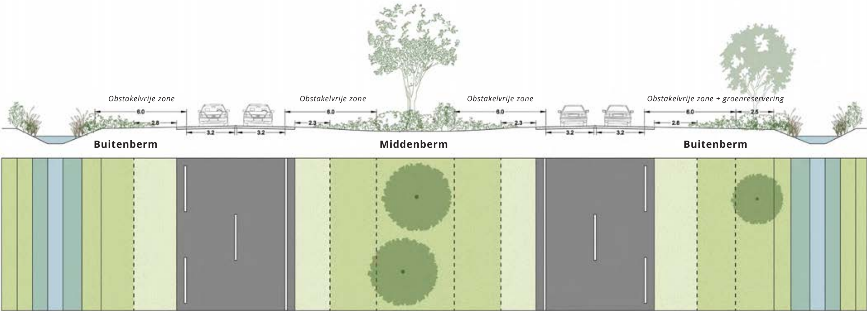
Principeprofiel binnen- en buitenberm Laan van Nieuw Land
