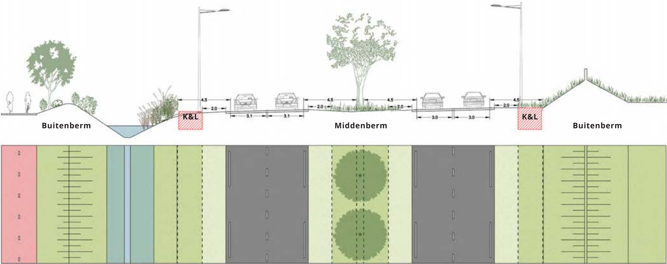
Principeprofiel binnen- en buitenberm Verlengde Westerdreef
