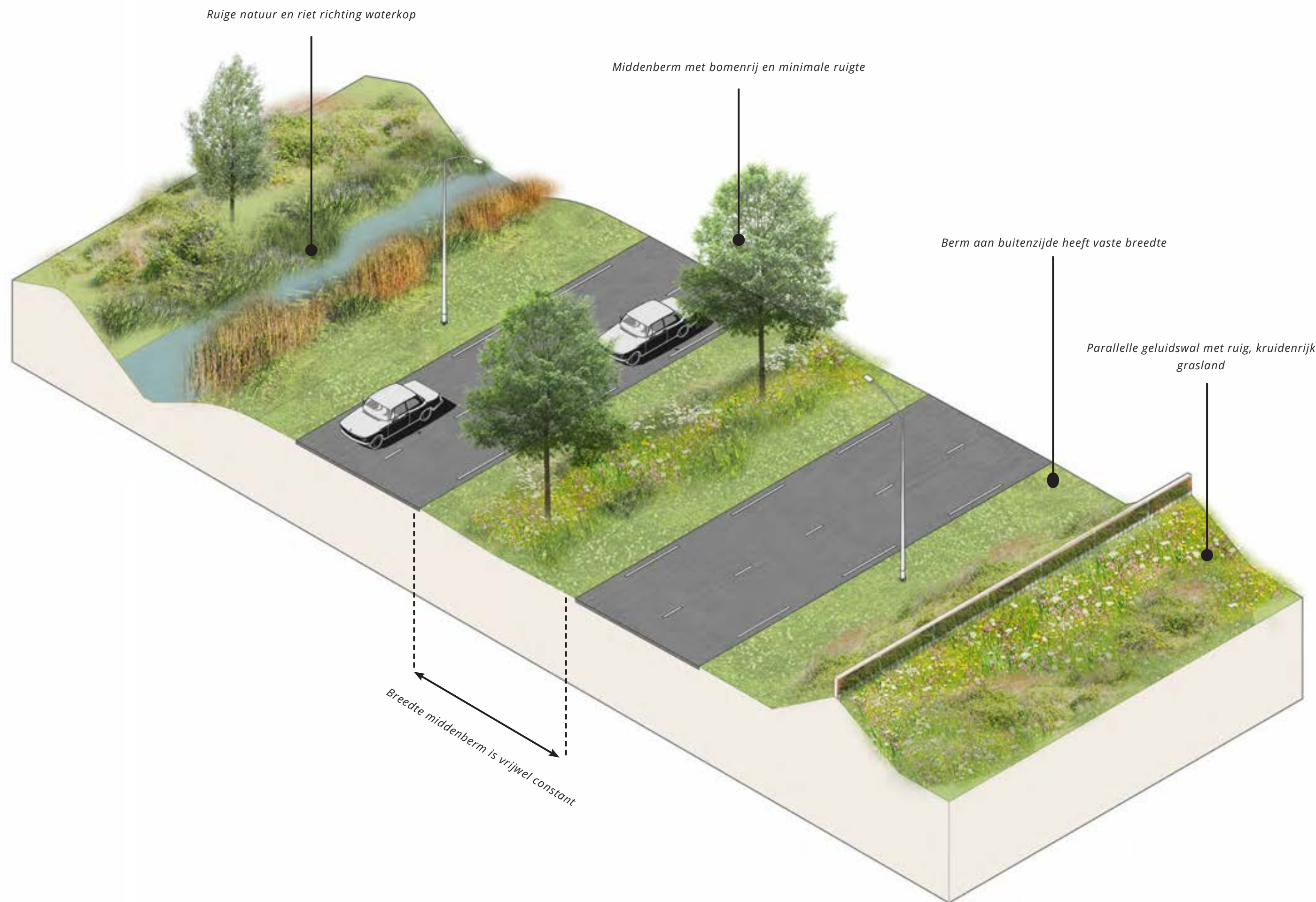
Principeprofiel binnen- en buitenberm Verlengde Westerdreef
