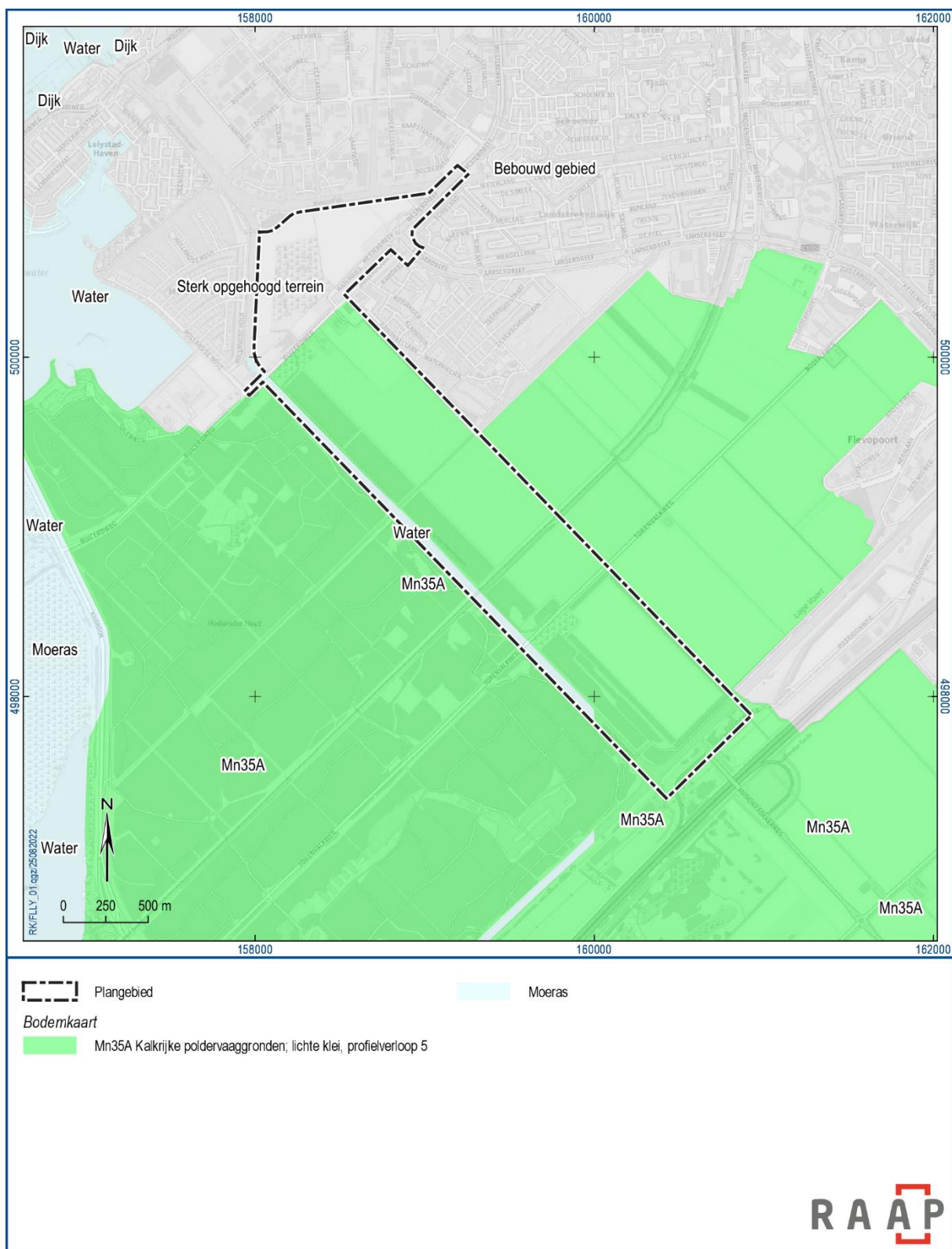
Figuur 7. Bodemkaart.
